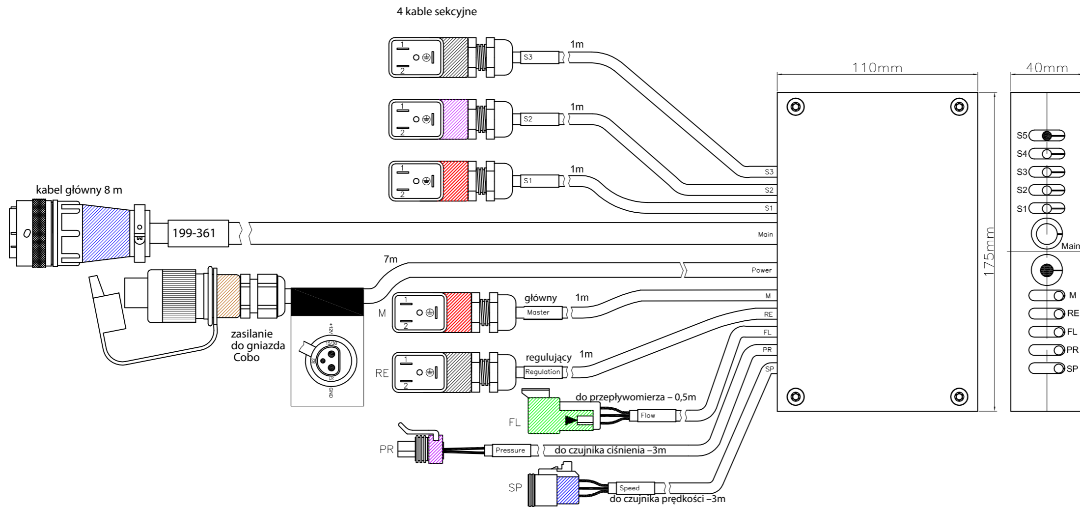
Połączenia wtyczki kabla głównego
